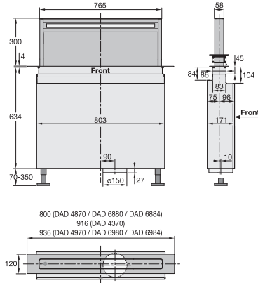
DAD 4370, DAD 4870, DAD 4970, DAD 6880, DAD 6980, Skizze
