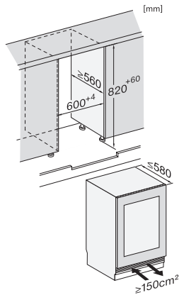
KWTUS7054F, KWTUS7055F, KWTUS7074F, KWTUS7096E, Built-under, Nischenmaß
