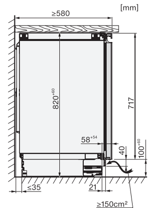
KWTUS7054F, KWTUS7055F, KWTUS7074F, Built-under, Seitenansicht
