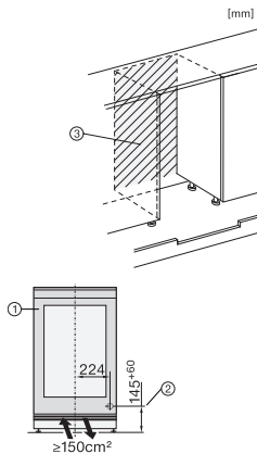
KWTUS7054F, KWTUS7055F, KWTUS7074F, KWTUS7096E, KWTUS7196E, Built-under, Installationsskizze (*Fußnote)
