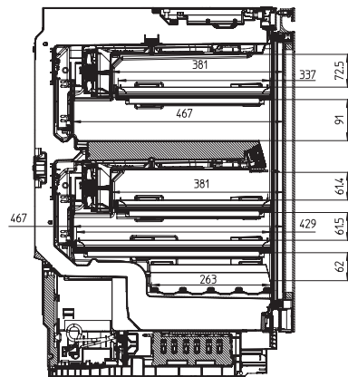
KWTUS7074F, Innenraummaße
