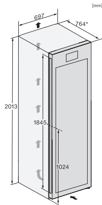
KWT4999F obsw, KWT4995F obsw, Rioja, Aufstellskizze
