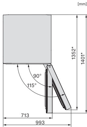
KWT4999F obsw, KWT4995F obsw, Rioja, Draufsicht
