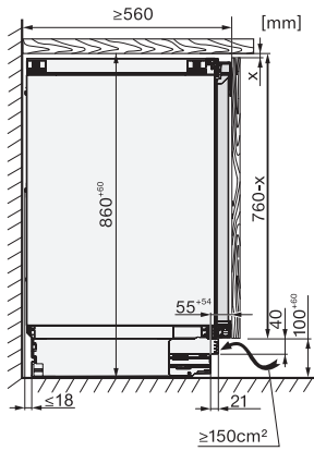
KU7135C, FNUS7140C, Built-under, Seitenansicht
