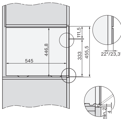
Seitenansicht DGC XL, Skizze A) 22 mm Glas, 23,3 mm Edelstahl
