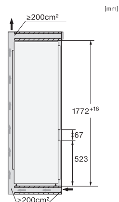
KF7731E, KF7731D, Seitenansicht
