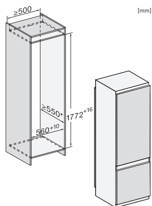
KF7731E, KF7731D, Einbau
