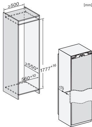
FNS7794D L, FNS7794D R, K7797C L, K7797C R, K7798C L, K7798C R, Einbau
