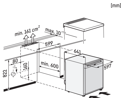
K4003D ws, K4002D ws, Aufstellskizze
