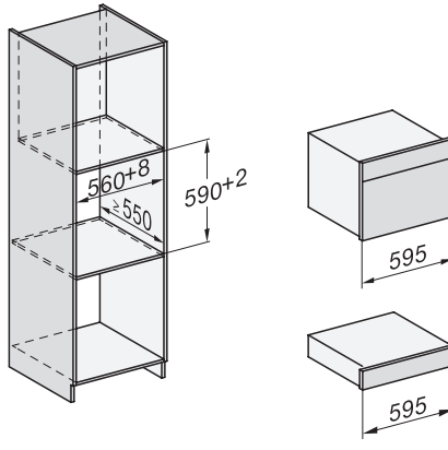
Einbau_DG_DGM_DGC_XL_ESW7x10_EVS7010 Skizze
