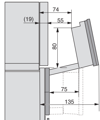
DGC7x4x Schwenkbereich der Blende, Skizze
