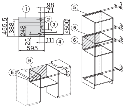
Einbau_DG_DGM_DGC_XL_ESW7x10_EVS7010 Skizze
