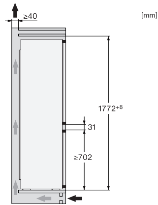
KFN7714F, KFNS7716FC, KD7714E, KD7724E, KDN7714E, KDN7724E Active, Seitenansicht
