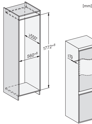
KFN7714F, KFNS7716FC, KD7714E, KD7724E, KDN7714E, KDN7724E Active, Einbau
