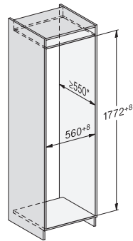
KFN7714F, KFNS7716FC, KD7714E, KD7724E, KDN7714E, KDN7724E Active, Einbau
