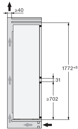
KFN7714F, KFNS7716FC, KD7714E, KD7724E, KDN7714E, KDN7724E Active, Seitenansicht
