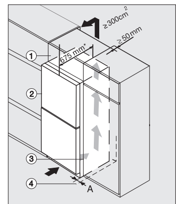
Freistehendes Kältegerät mit Metallfront in eine Küchenzeile integrieren, edt/cs, ws, bst, el
