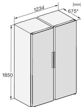
KS4383DD, KS4383ED, KS4887DD, FNS4382D, FNS4382E, FNS4882D, Aufstellskizze, Side-by-Side
