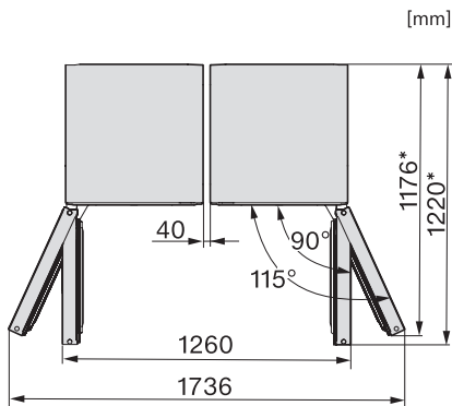
KS4887DD, FNS4882D, Draufsicht, Side-by-Side
