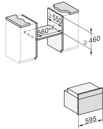
Einbau H7000 M Unterbau, Skizze
