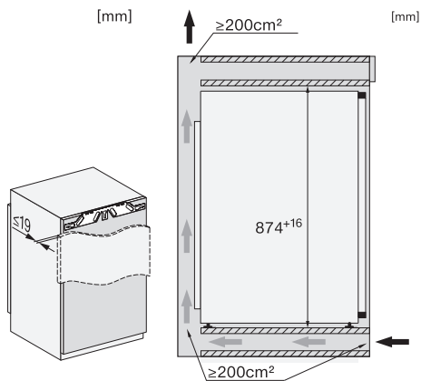
FNS7140B, FNS7140C, FNS7140D, FNS7140E, Einbau
