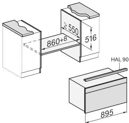
Einbau H7000 90 Unterbau, Skizze
