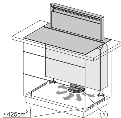
DAD4840, DAD4940 - DUP150, Einbauvariante 1, Skizze, Ausströmpfeile, Positionsnummer
