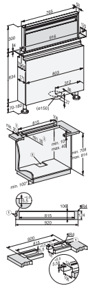
DAD4840, Skizze
